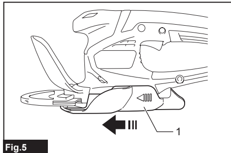
► 1. Collecteur d'herbes
